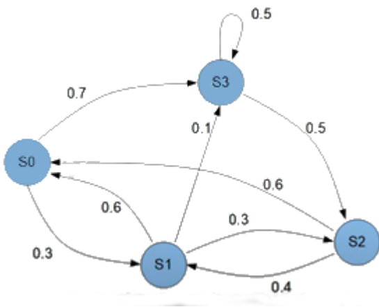
Figure 20 : Chaînes de MARKOV
